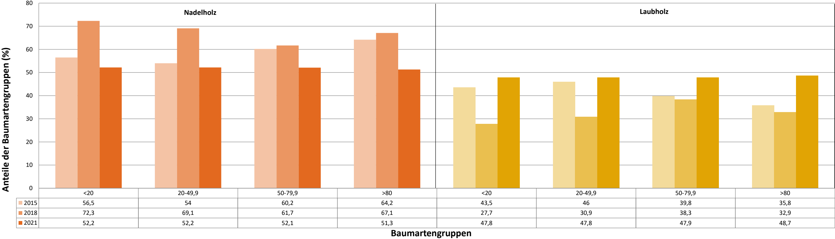
Anteile der Baumartengruppen in verschiedenen Höhenstufen für die Hegegemeinschaft 131 - Hg IX Bad Aibling Süd/Dettendf. (Landkreis Rosenheim)
